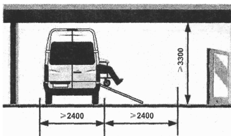
Рисунок Д.6. Автостоянки
